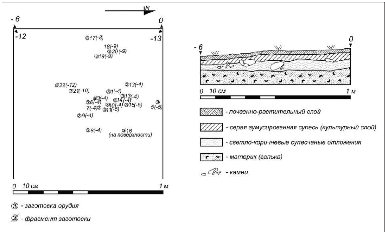
Рис. 2. План расположения находок и стратиграфия Иганджинского клада
