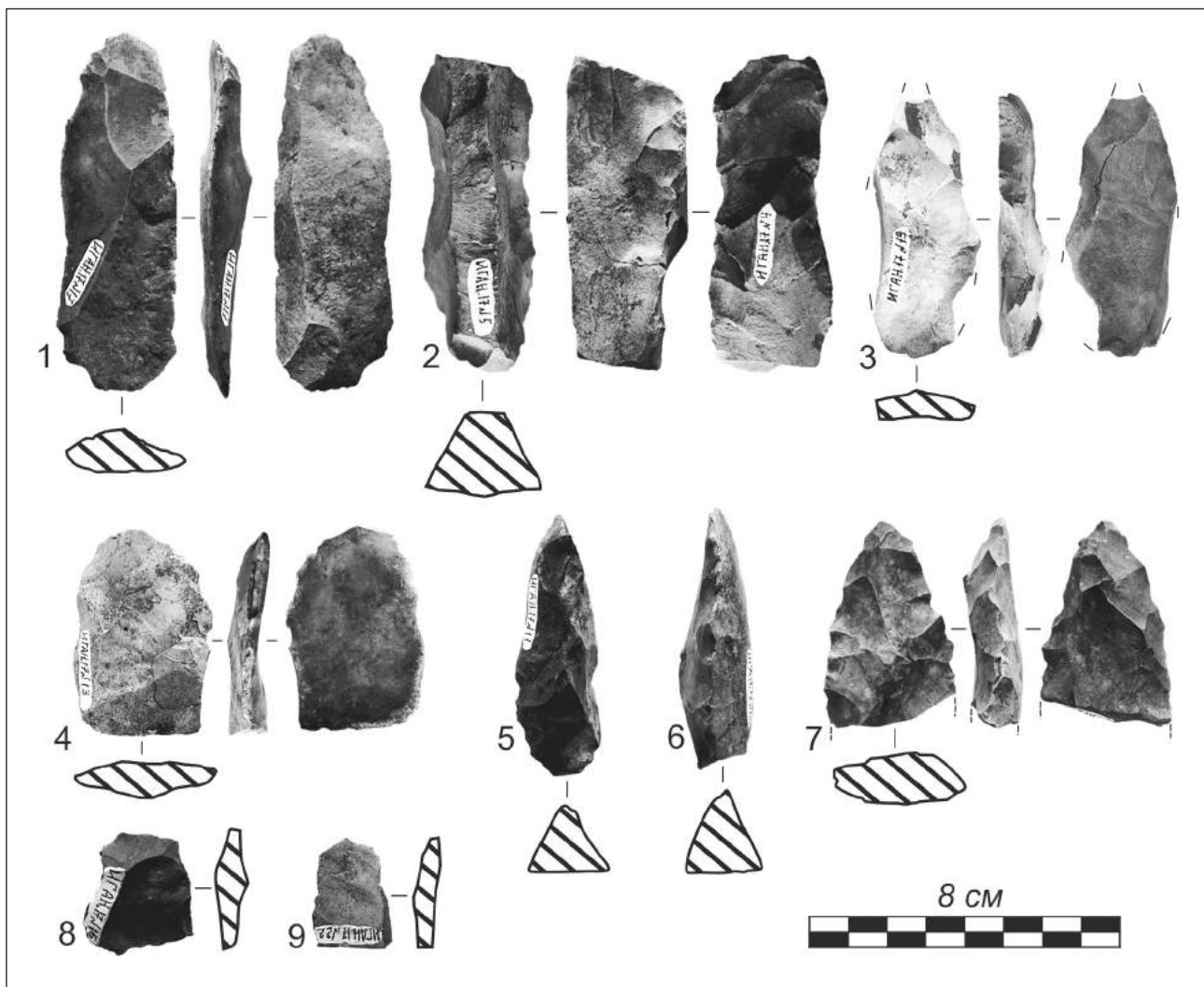
Рис. 4. Иганджинский клад (1 – заготовка орудия на пластине, 2 – заготовка с трапециевидным сечением, 3 – фрагментированная заготовка, 4 – заготовка на отщепе, 5-6 – трехгранные напильниковидные заготовки, 7 – фрагмент заготовки, острие, 8-9 – фрагменты заготовок орудий)
