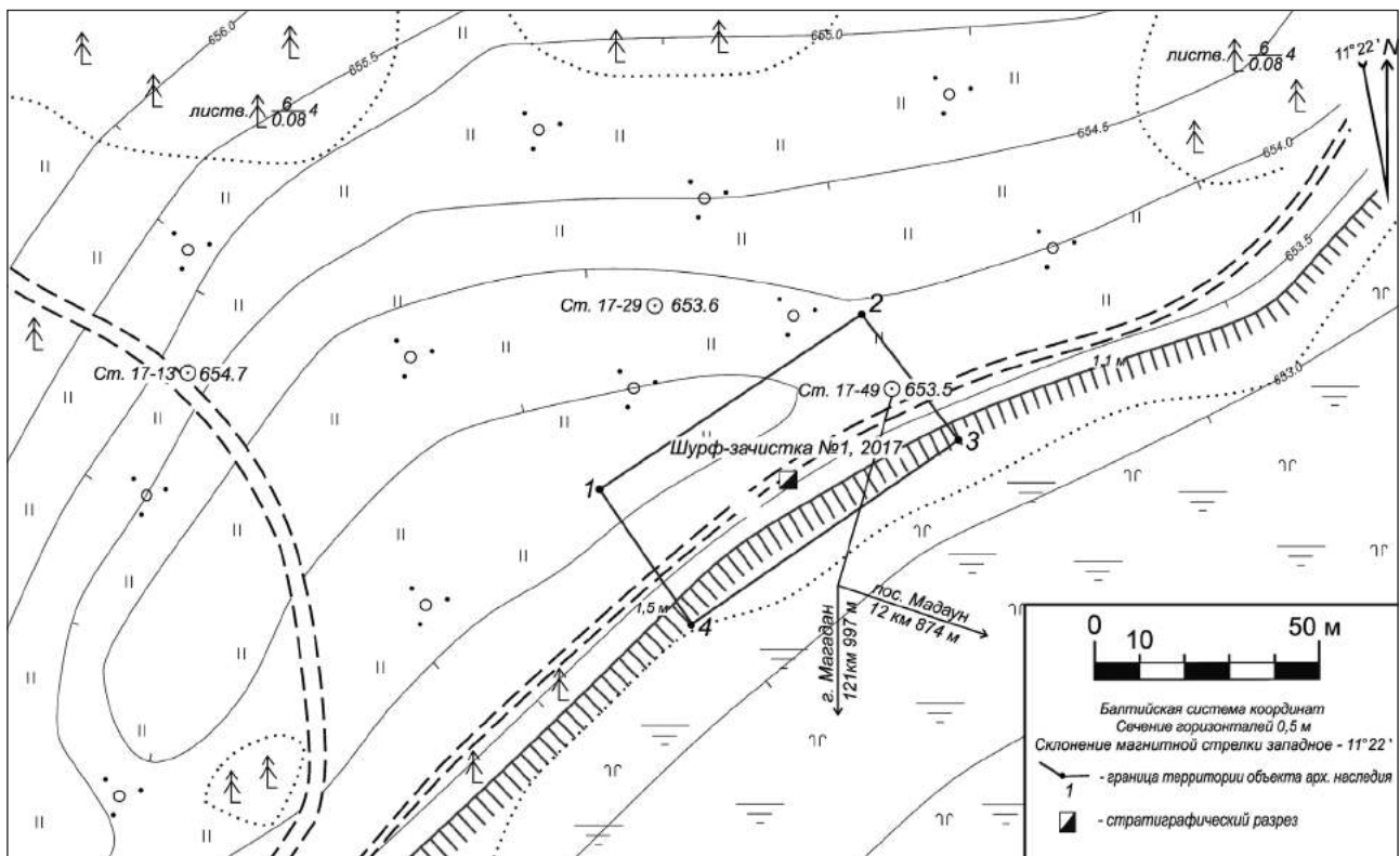
Рис. 1. Топографический план месторасположения Иганджинского клада (Магаданская обл.). М. 1 : 1000
